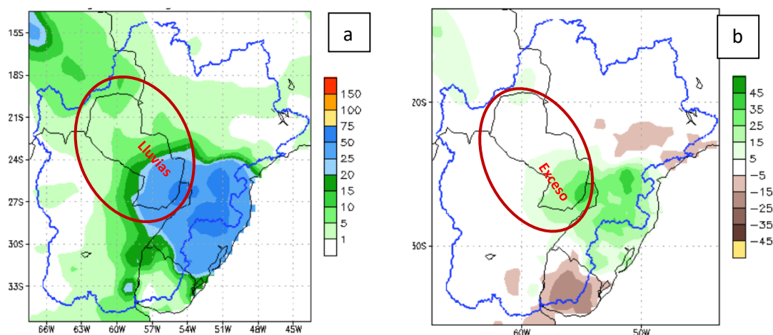
Figura 1: a) Cantidad de lluvia prevista (en mm) desde el 06 al 12 de agosto. b) Anomalía de lluvia acumulada (en mm) desde el 06 al 12 de agosto. En él se pueden determinar las zonas con posibles excesos (verde) o déficits (marrón) de lluvias previstas para esas fechas. Fuente: NOAA.
