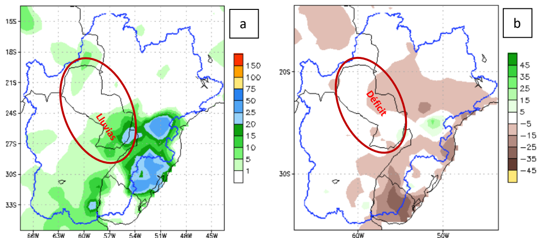
Figura 2: a) Cantidad de lluvia prevista (en mm) desde el 13 al 19 de agosto. b) Anomalía de lluvia acumulada desde el 13 al 19 de agosto. En él se pueden determinar las zonas con posibles excesos (verde) o déficits (marrón) de lluvias previstas para esas fechas. Fuente: NOAA.
