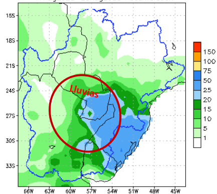
Figura 2: a) Cantidad de lluvia prevista (en mm) desde el 17 al 23 de agosto . b) Anomalía de lluvia acumulada desde el 17 al 23 de agosto . En él se pueden determinar las zonas con posibles excesos (verde) o déficits (marrón) de lluvias previstas para esas fechas. Fuente: NOAA.
