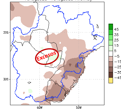
Figura 1: a) Cantidad de lluvia prevista (en mm) desde el 10 al 16 de agosto . b) Anomalía de lluvia acumulada (en mm) desde el 10 al 16 de agosto . En él se pueden determinar las zonas con posibles excesos (verde) o déficits (marrón) de lluvias previstas para esas fechas. Fuente: NOAA.
