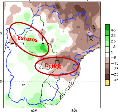
Figura 2: a) Cantidad de lluvia prevista (en mm) desde el 18 al 24 de mayo . b) Anomalía de lluvia acumulada desde el 18 al 24 de mayo . En él se pueden determinar las zonas con posibles excesos (verde) o déficits (marrón) de lluvias previstas para esas fechas. Fuente: NOAA.
