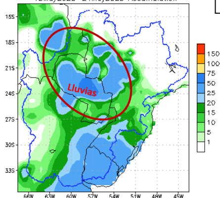
Figura 2: a) Cantidad de lluvia prevista (en mm) desde el 18 al 24 de mayo . b) Anomalía de lluvia acumulada desde el 18 al 24 de mayo . En él se pueden determinar las zonas con posibles excesos (verde) o déficits (marrón) de lluvias previstas para esas fechas. Fuente: NOAA.
