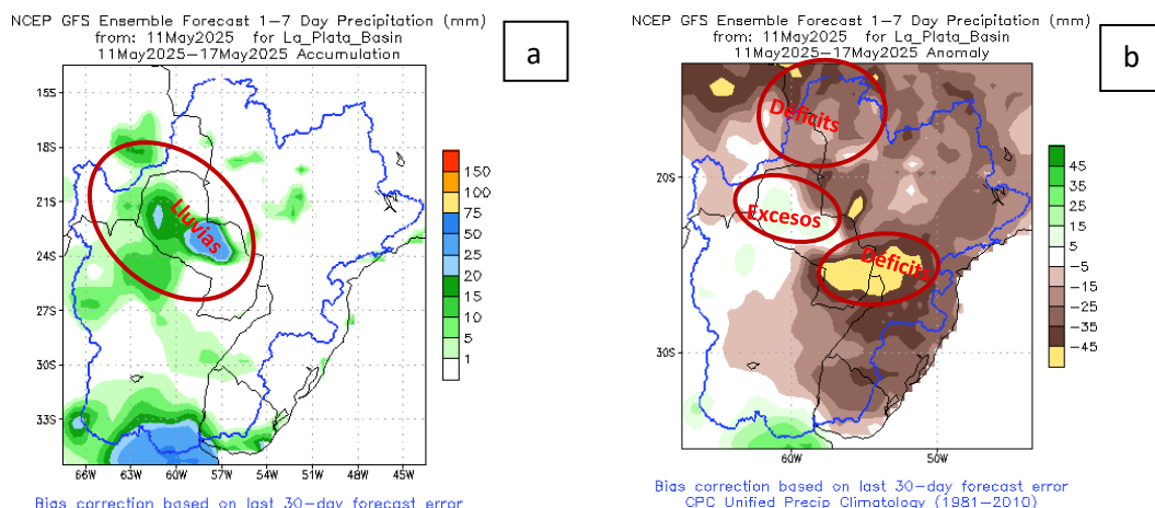
Figura 1: a) Cantidad de lluvia prevista (en mm) desde el 11 al 17 de mayo . b) Anomalía de lluvia acumulada (en mm) desde el 11 al 17 de mayo . En él se pueden determinar las zonas con posibles excesos (verde) o déficits (marrón) de lluvias previstas para esas fechas. Fuente: NOAA.
