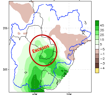
Figura 1: a) Cantidad de lluvia prevista (en mm) desde el 17 al 23 de agosto . b) Anomalia de lluvia acumulada (en mm) desde el 17 al 23 de agosto . En él se pueden determinar las zonas con posibles excesos (verde) o déficits (marrón) de lluvias previstas para esas fechas. Fuente: NOAA.
