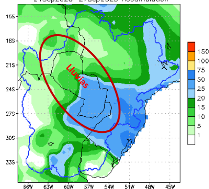
Figura 1: a) Cantidad de lluvia prevista (en mm) desde el 21 al 27 de setiembre . b) Anomalía de lluvia acumulada (en mm) desde el 21 al 27 de setiembre . En él se pueden determinar las zonas con posibles excesos (verde) o déficits (marrón) de lluvias previstas para esas fechas. Fuente: NOAA.
