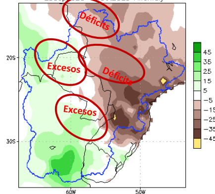
Figura 2: a) Cantidad de lluvia prevista (en mm) desde el 28 de septiembre al 01 de octubre . b) Anomalía de lluvia acumulada desde el 28 de septiembre al 01 de octubre . En él se pueden determinar las zonas con posibles excesos (verde) o déficits (marrón) de lluvias previstas para esas fechas. Fuente: NOAA.
