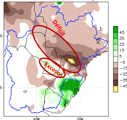
Figura 2: a) Cantidad de lluvia prevista (en mm) desde el 02 al 08 de junio. b) Anomalía de lluvia acumulada desde el 02 al 08 de junio. En él se pueden determinar las zonas con posibles excesos (verde) o déficits (marrón) de lluvias previstas para esas fechas. Fuente: NOAA.
