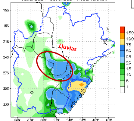
Figura 2: a) Cantidad de lluvia prevista (en mm) desde el 02 al 08 de junio. b) Anomalía de lluvia acumulada desde el 02 al 08 de junio. En él se pueden determinar las zonas con posibles excesos (verde) o déficits (marrón) de lluvias previstas para esas fechas. Fuente: NOAA.
