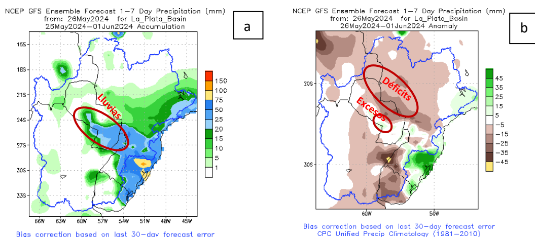
Figura 1: a) Cantidad de lluvia prevista (en mm) desde el 26 de mayo al 01 de junio. b) Anomalía de lluvia acumulada (en mm) desde el 26 de mayo al 01 de junio. En él se pueden determinar las zonas con posibles excesos (verde) o déficits (marrón) de lluvias previstas para esas fechas. Fuente: NOAA.
