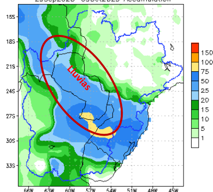
Figura 1: a) Cantidad de lluvia prevista (en mm) desde el 29 de setiembre al 05 de octubre . b) Anomalía de lluvia acumulada (en mm) desde el 29 de setiembre al 05 de octubre . En él se pueden determinar las zonas con posibles excesos (verde) o déficits (marrón) de lluvias previstas para esas fechas. Fuente: NOAA.
