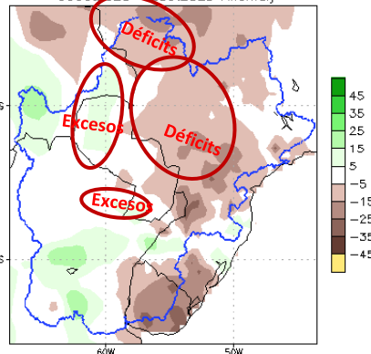
Figura 2: a) Cantidad de lluvia prevista (en mm) desde el 08 al 12 de octubre . b) Anomalía de lluvia acumulada desde el 08 al 12 de octubre . En él se pueden determinar las zonas con posibles excesos (verde) o déficits (marrón) de lluvias previstas para esas fechas. Fuente: NOAA.
