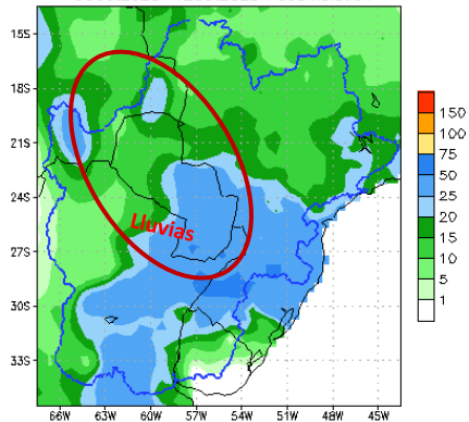
Figura 2: a) Cantidad de lluvia prevista (en mm) desde el 08 al 12 de octubre . b) Anomalía de lluvia acumulada desde el 08 al 12 de octubre . En él se pueden determinar las zonas con posibles excesos (verde) o déficits (marrón) de lluvias previstas para esas fechas. Fuente: NOAA.
